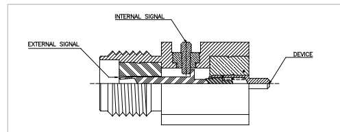
JSCF-7 (SMA straight Side TYPE) (SMA CONN. 구조를 응용하여 Switching Jack을 구현)
