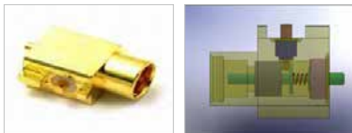
JSCF-9 (MMCX Straight Side TYPE) (MMCX CONN. 구조를 응용하여 Switching Jack을 구현)
