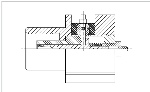
JSCF-5 & JSCF-6 (MCX straight Side TYPE)
